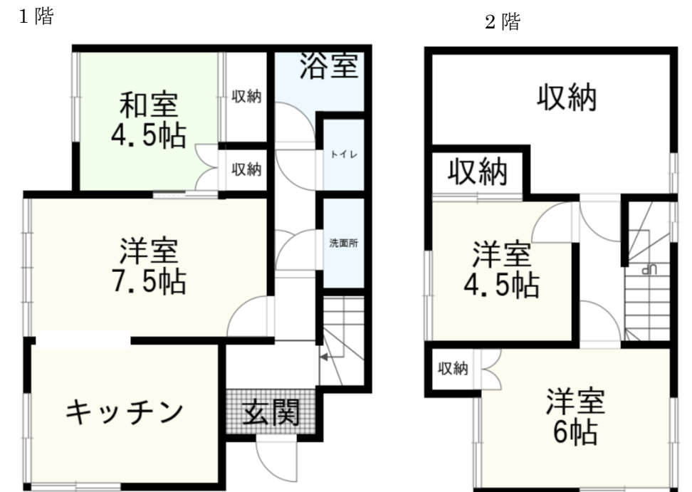
間取り図
