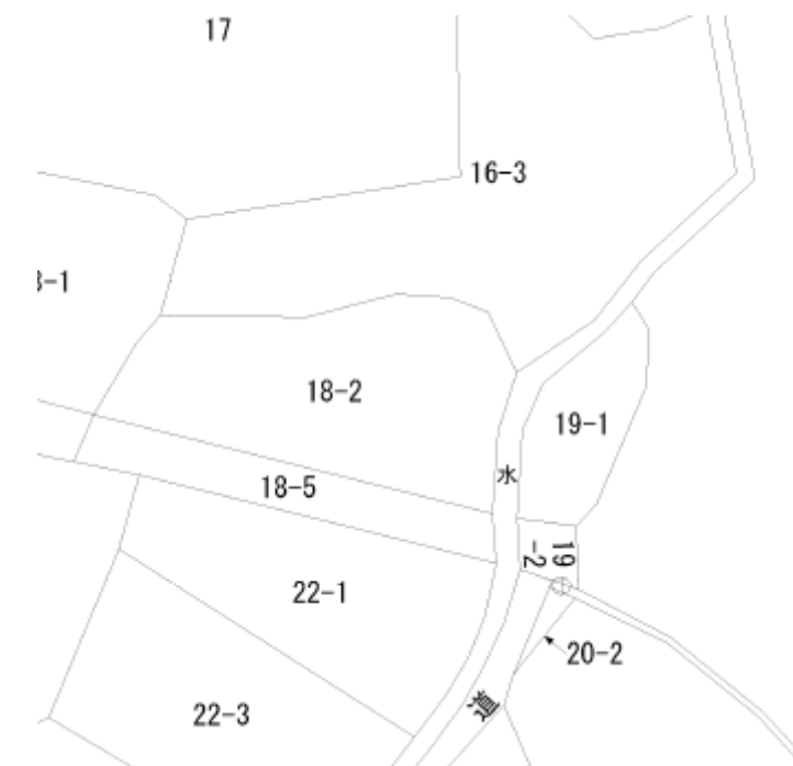
区画図 (地形)
