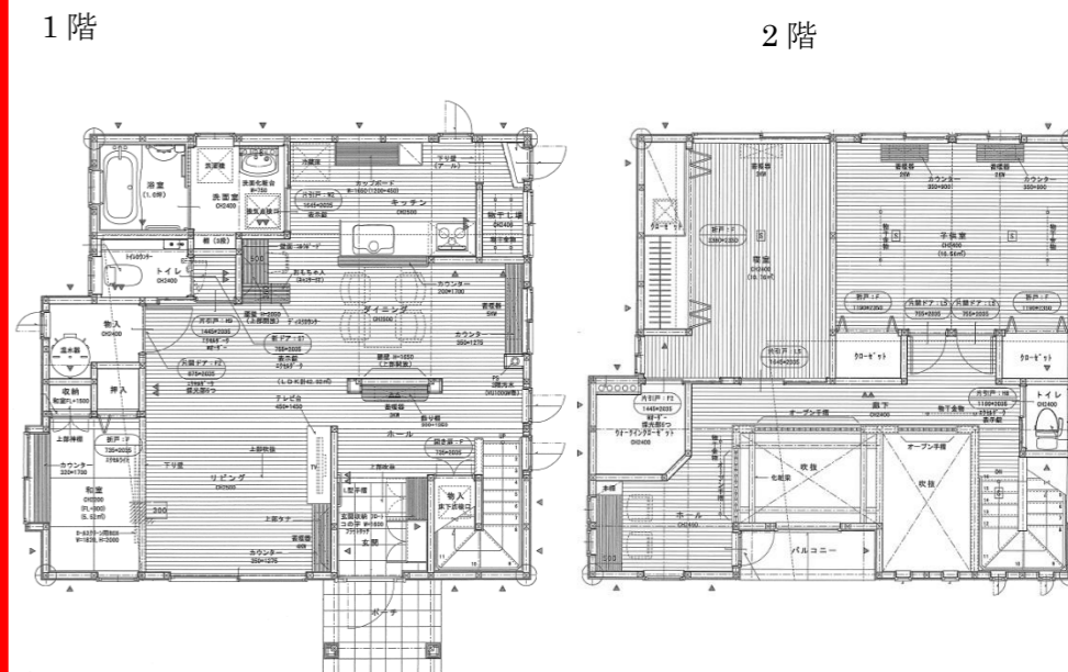
間取り図
