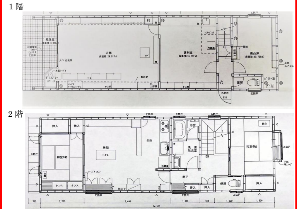
間取り図
